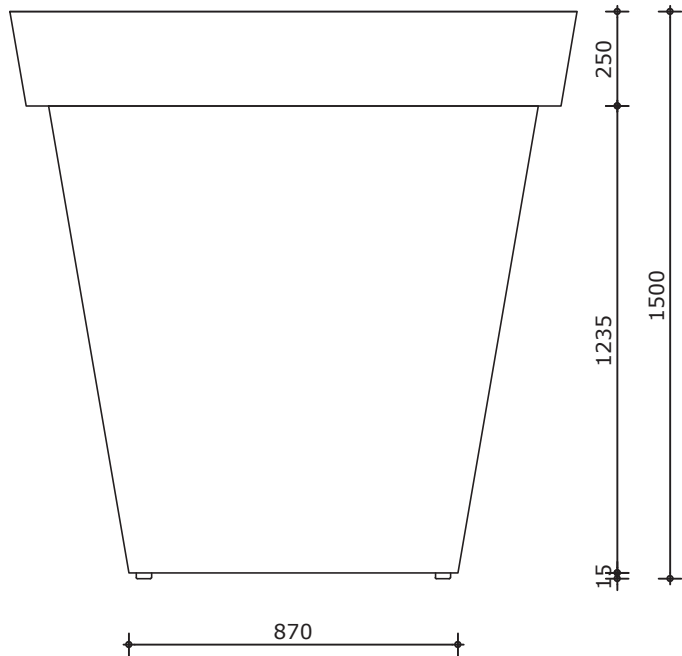
Voorraanzicht
