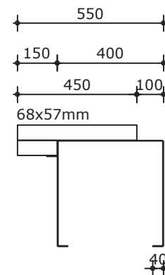
Verticale doorsnede
