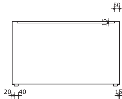
Verticale doorsnede
