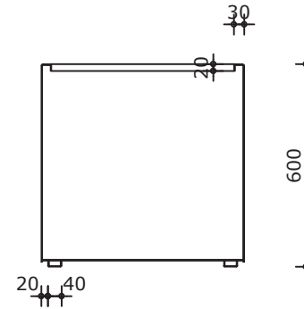
Verticale doorsnede
