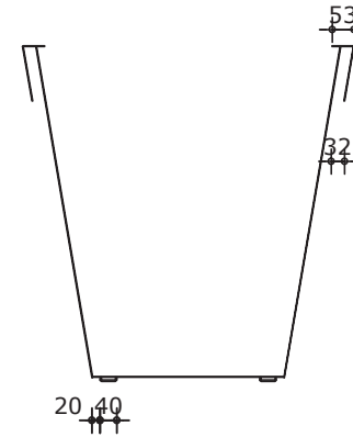
Doorsnede
