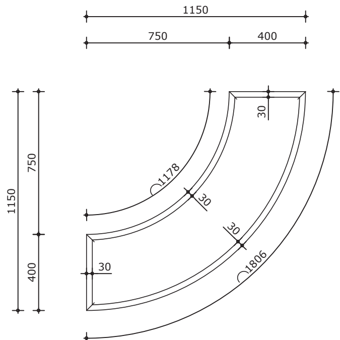
Bovenaanzicht
