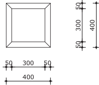
Bovenaanzicht
