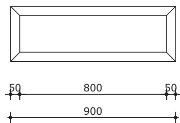
Bovenaanzicht
