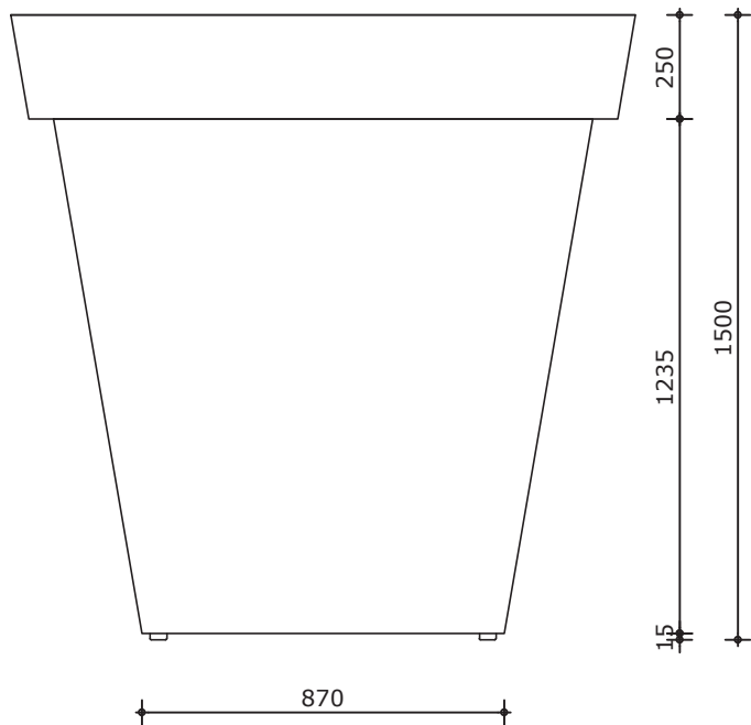
Voorraanzicht
