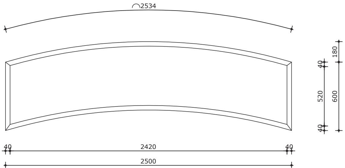
Bovenaanzicht
