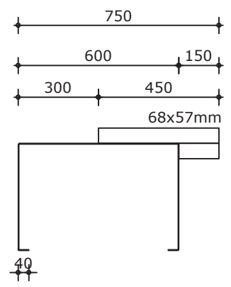
Verticale doorsnede
