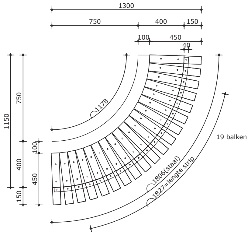
Bovenaanzicht
