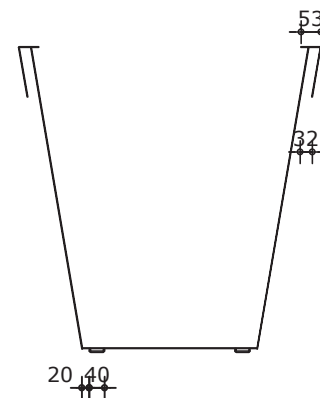
Doorsnede
