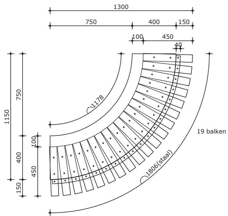
Bovenaanzicht
