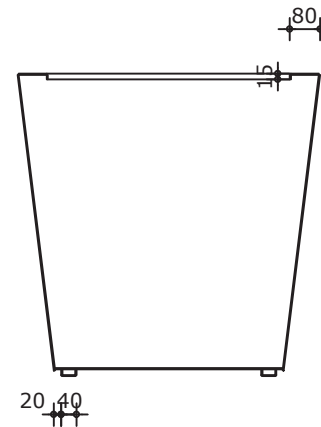
Verticale doorsnede
