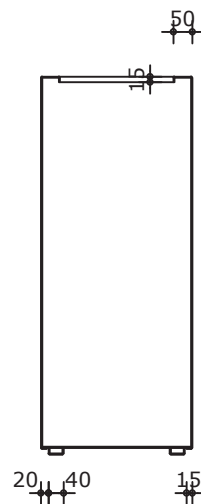
Verticale doorsnede
