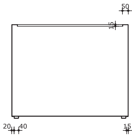
Verticale doorsnede
