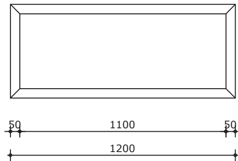
Bovenaanzicht
