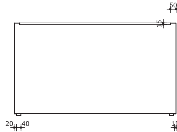
Verticale doorsnede
