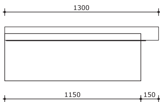
Vooraanzicht
