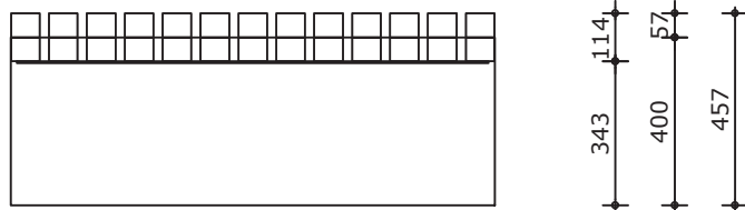
Voorraanzicht
