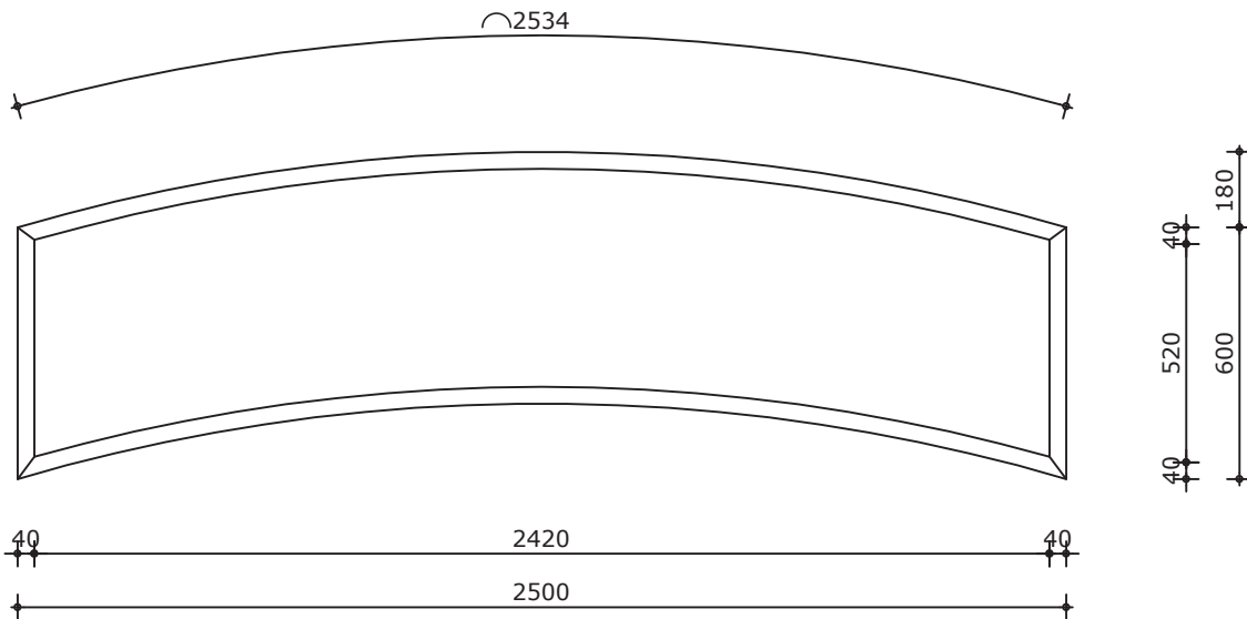
Bovenaanzicht
