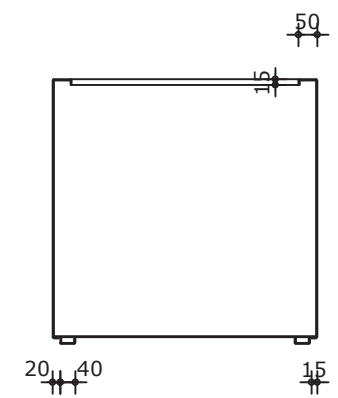
Verticale doorsnede
