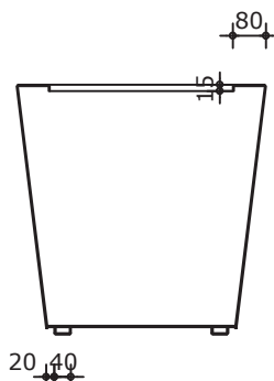
Verticale doorsnede
