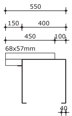
Verticale doorsnede
