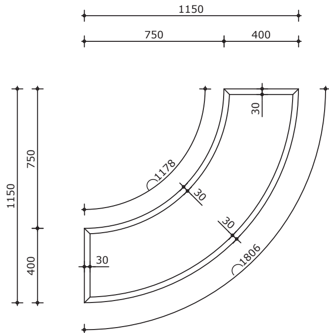
Bovenaanzicht
