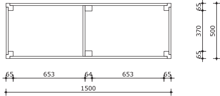
Bovenaanzicht
