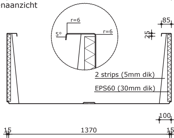
Doorsnede
