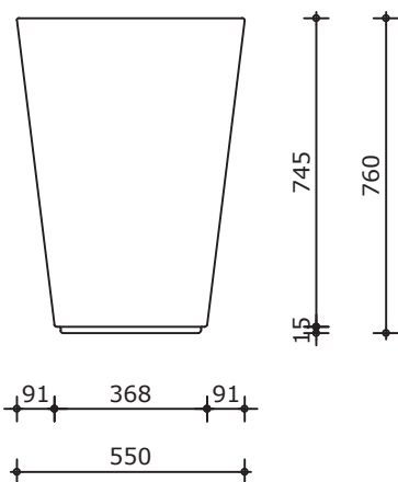
Vooraanzicht
