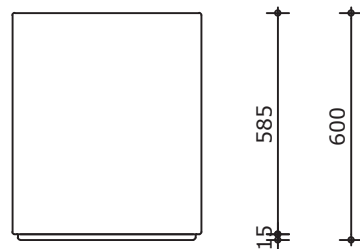
Vooraanzicht
