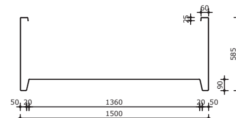
Langsdoorsnede
