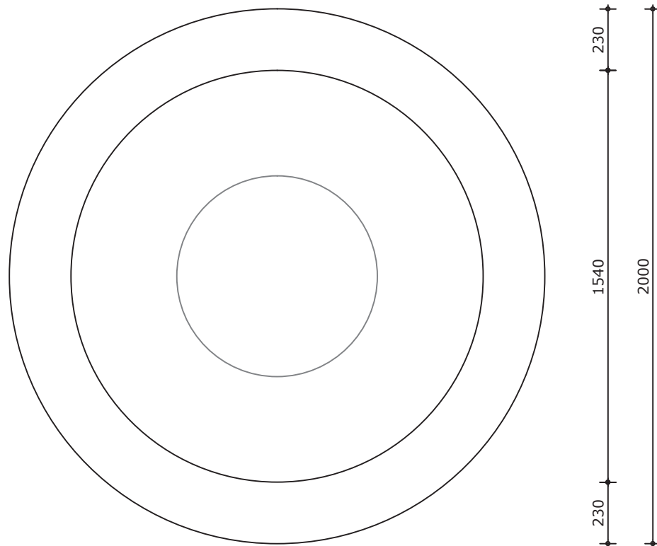
Bovenaanzicht
