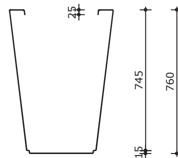
Doorsnede
