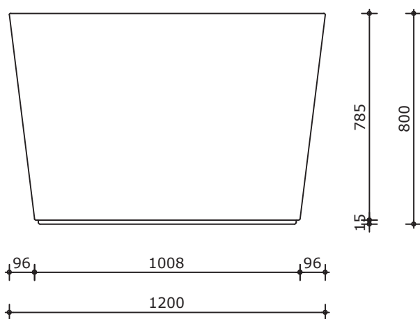
Vooraanzicht
