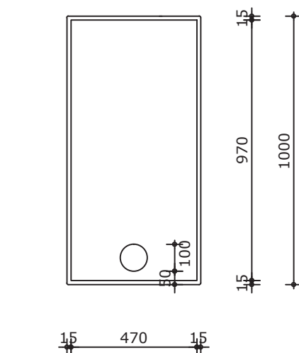
Onderaanzicht
