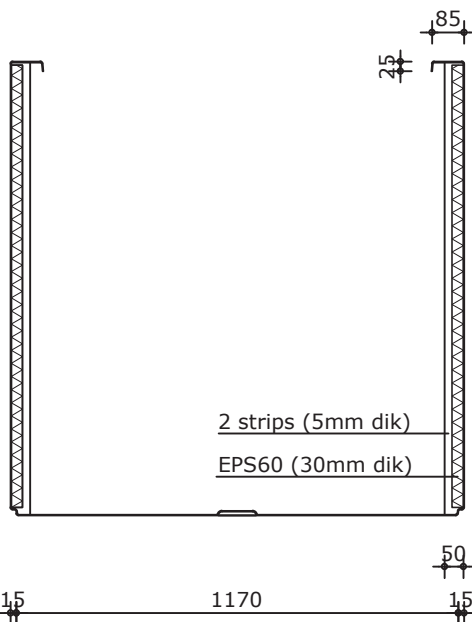
Doorsnede
