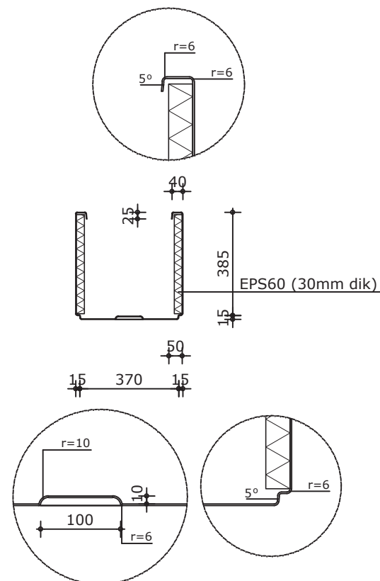
Doorsnede
