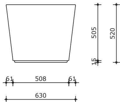
Vooraanzicht
