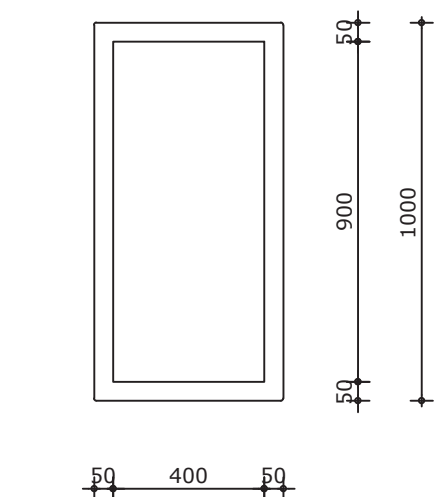
Bovenaanzicht
