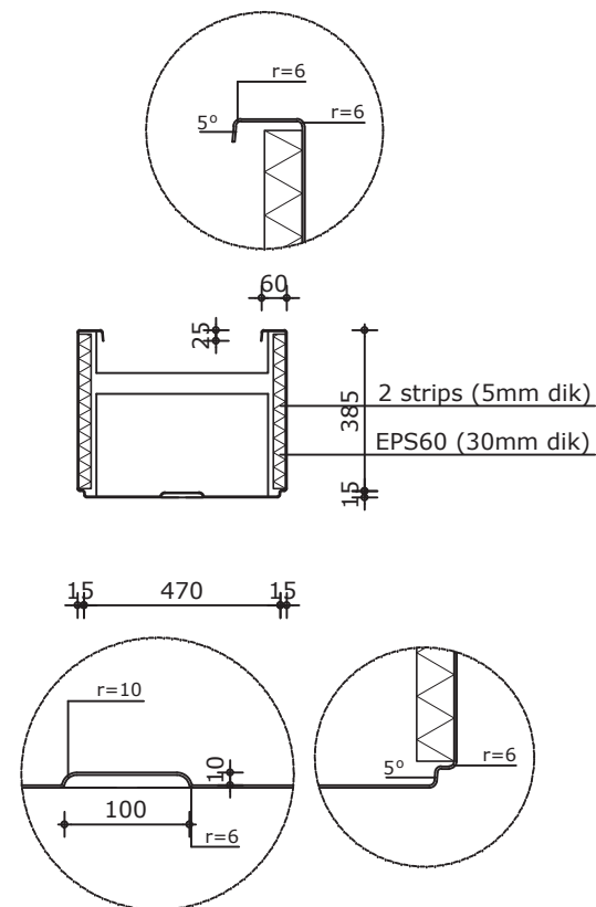
Doorsnede
