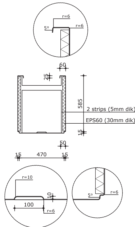
Doorsnede
