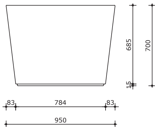
Vooraanzicht
