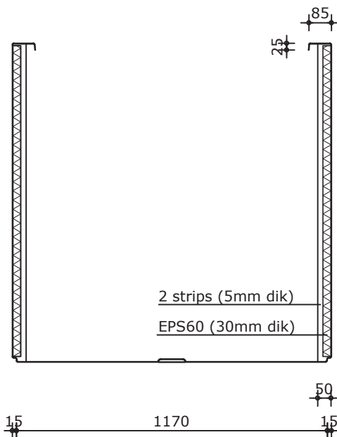
Doorsnede
