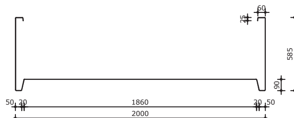
Langsdoorsnede
