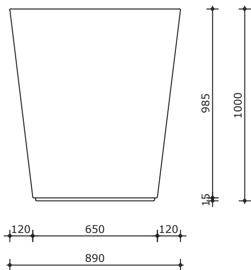
Vooraanzicht
