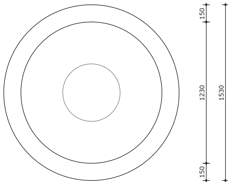
Bovenaanzicht
