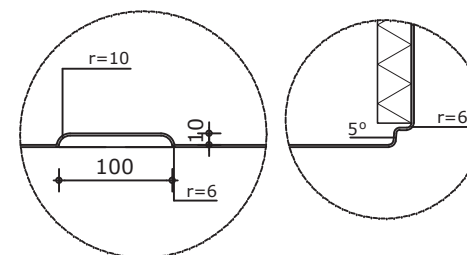
Doorsnede
