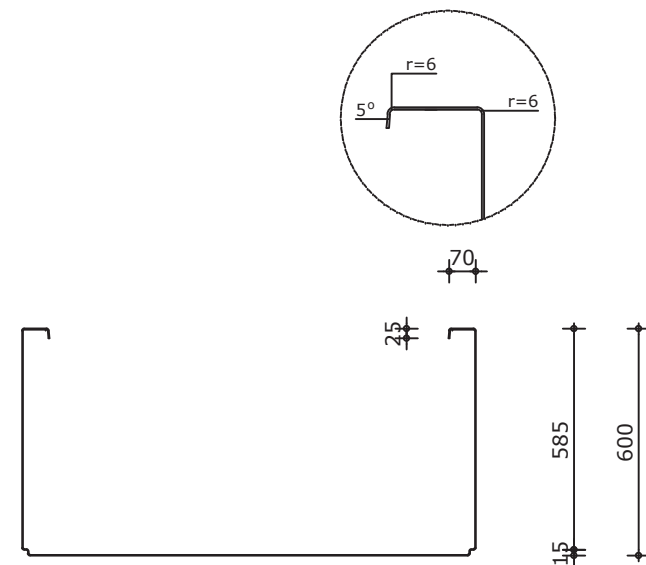
Doorsnede
