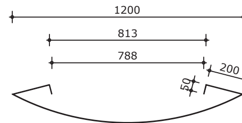
Doorsnede
