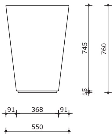
Vooraanzicht
