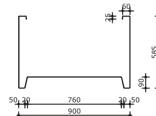
Langsdoorsnede
