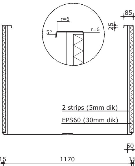
Bovenaanzicht
