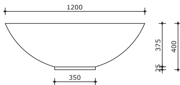
Vooraanzicht
