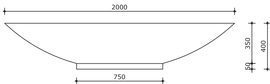
Vooraanzicht
