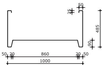
Langsdoorsnede
