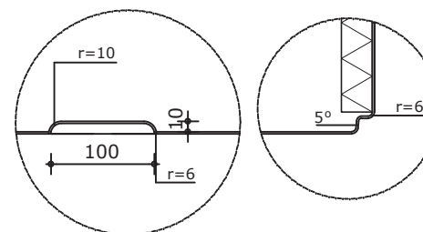
Doorsnede
