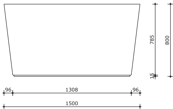
Vooraanzicht
