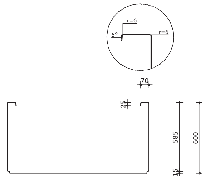
Doorsnede
