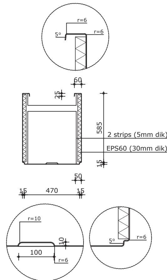
Doorsnede
