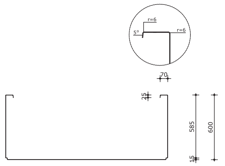
Doorsnede
