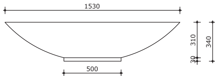
Vooraanzicht
