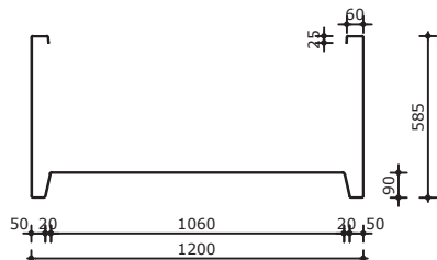
Langsdoorsnede
