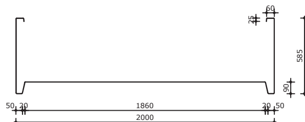
Langsdoorsnede
